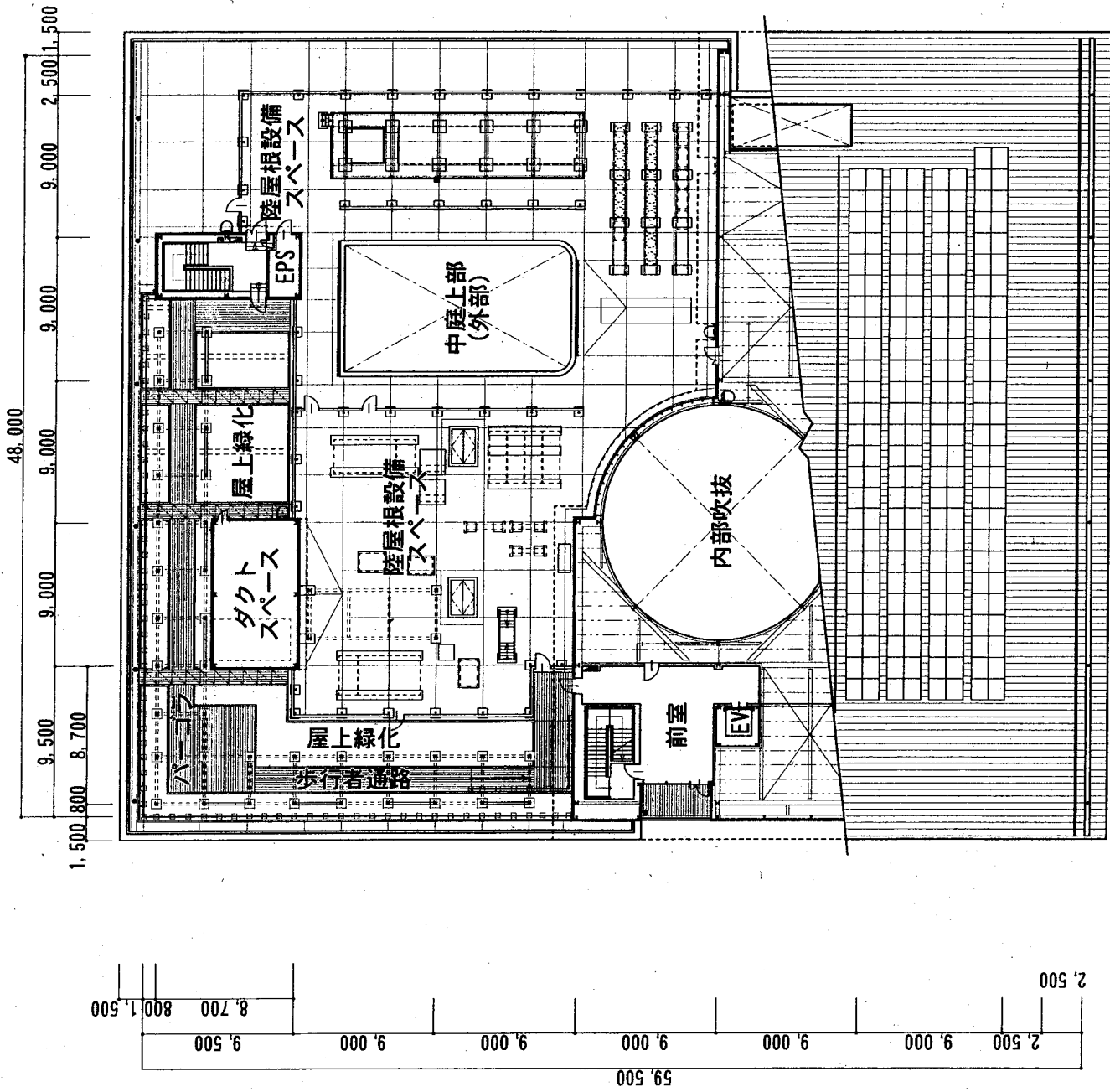
(仮) 新図書館複合施設建設工事 (建築工事)
